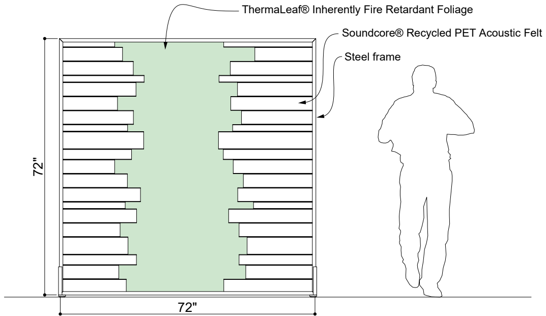
② ELEVATION 2
