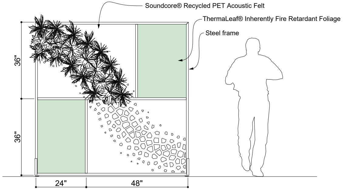
① ELEVATION 1
